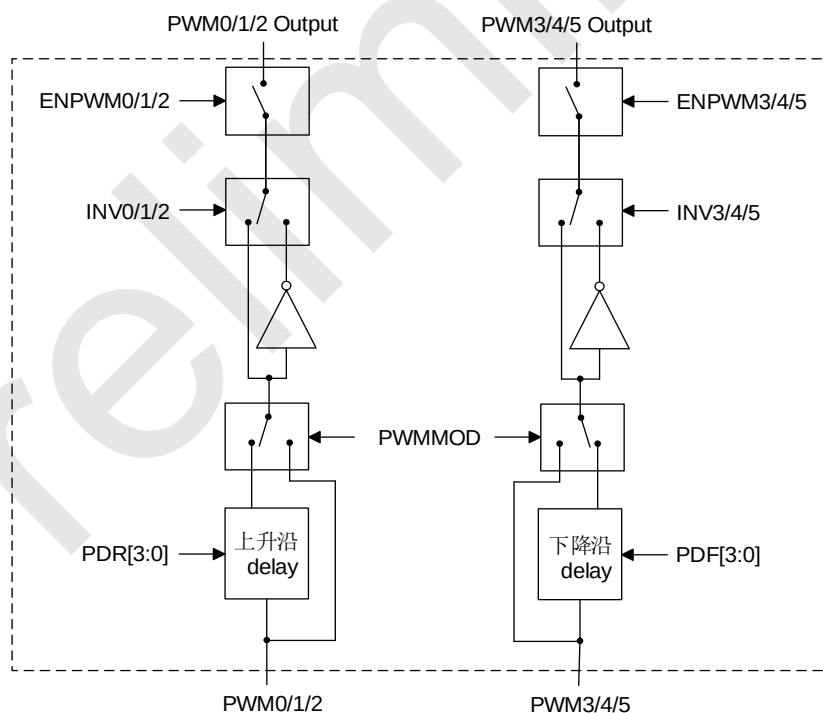
SC92R348 PWM 互补模式框图
