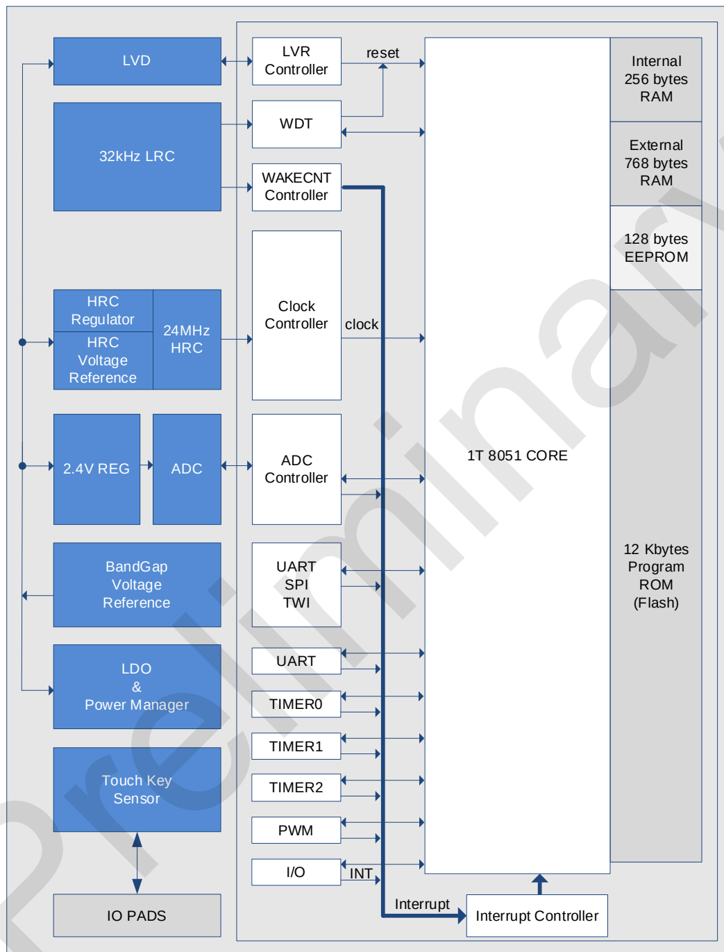
SC92R348 BLOCK DIAGRAM
