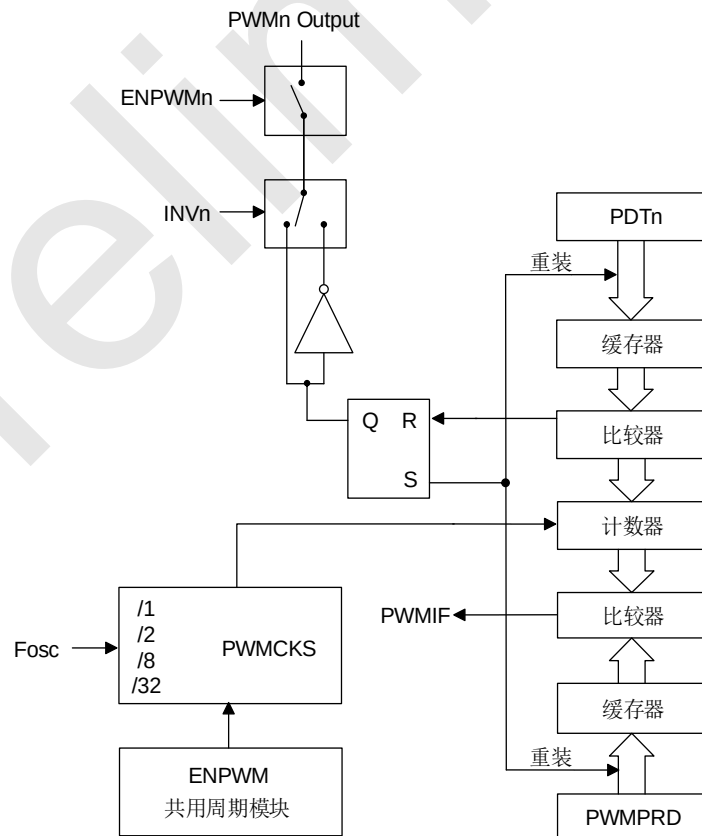
SC92R348 PWM 独立模式框图
