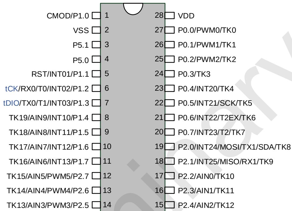
SOP28/TSSOP28 管脚配置图
