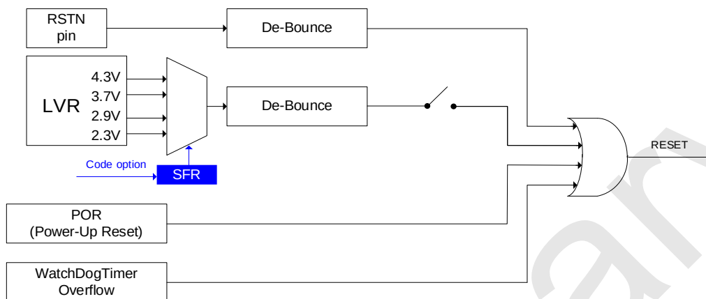
SC92R348 复位电路图
