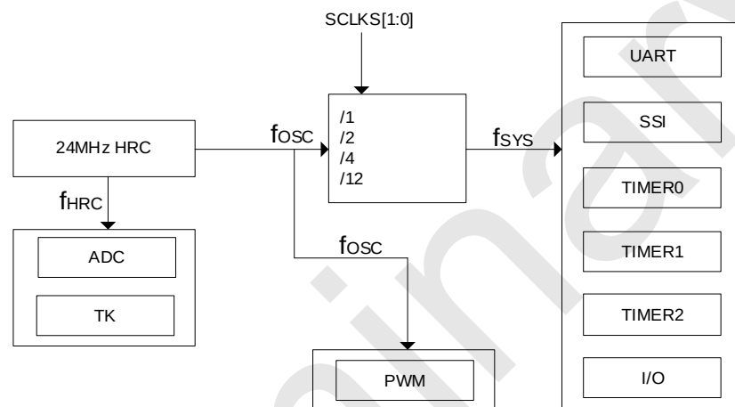
SC92R348 内部时钟关系
