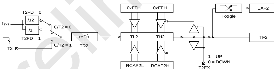
模式 1: 16 位自动重载 DCEN = 1
