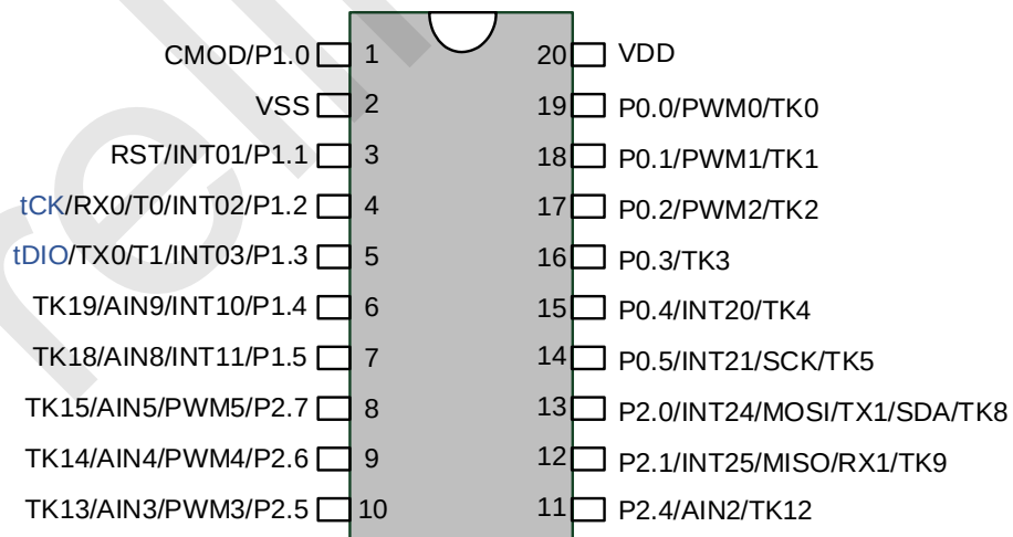
SOP20/TSSOP20 管脚配置图
