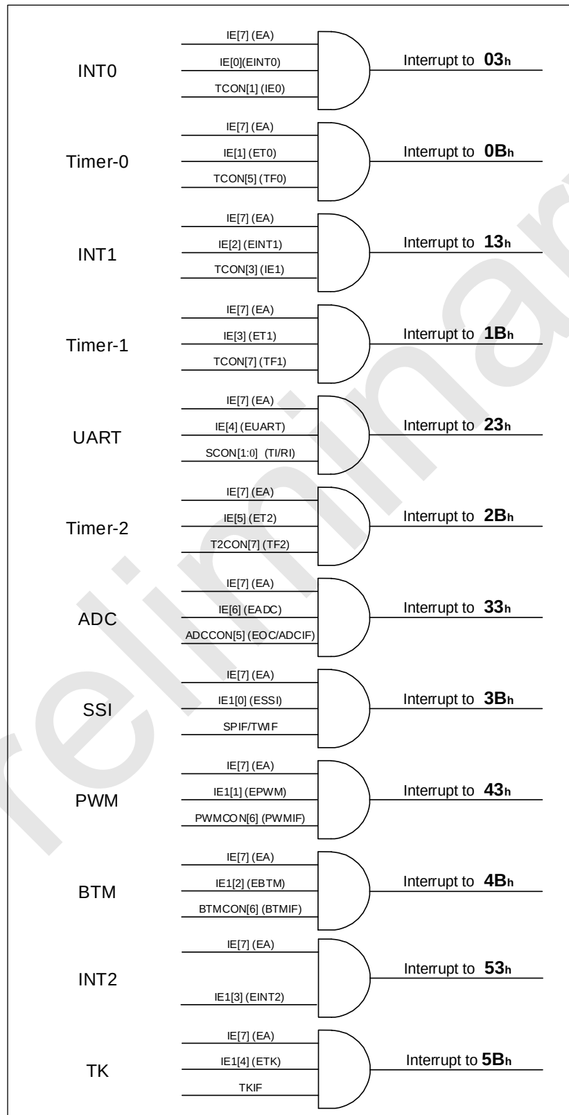
SC92R348 中断结构和向量
