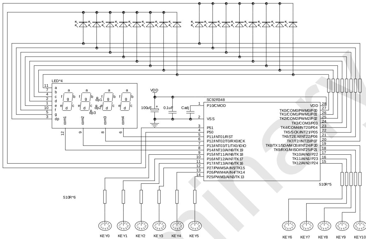
SC92R348 Touch Key 应用电路图
