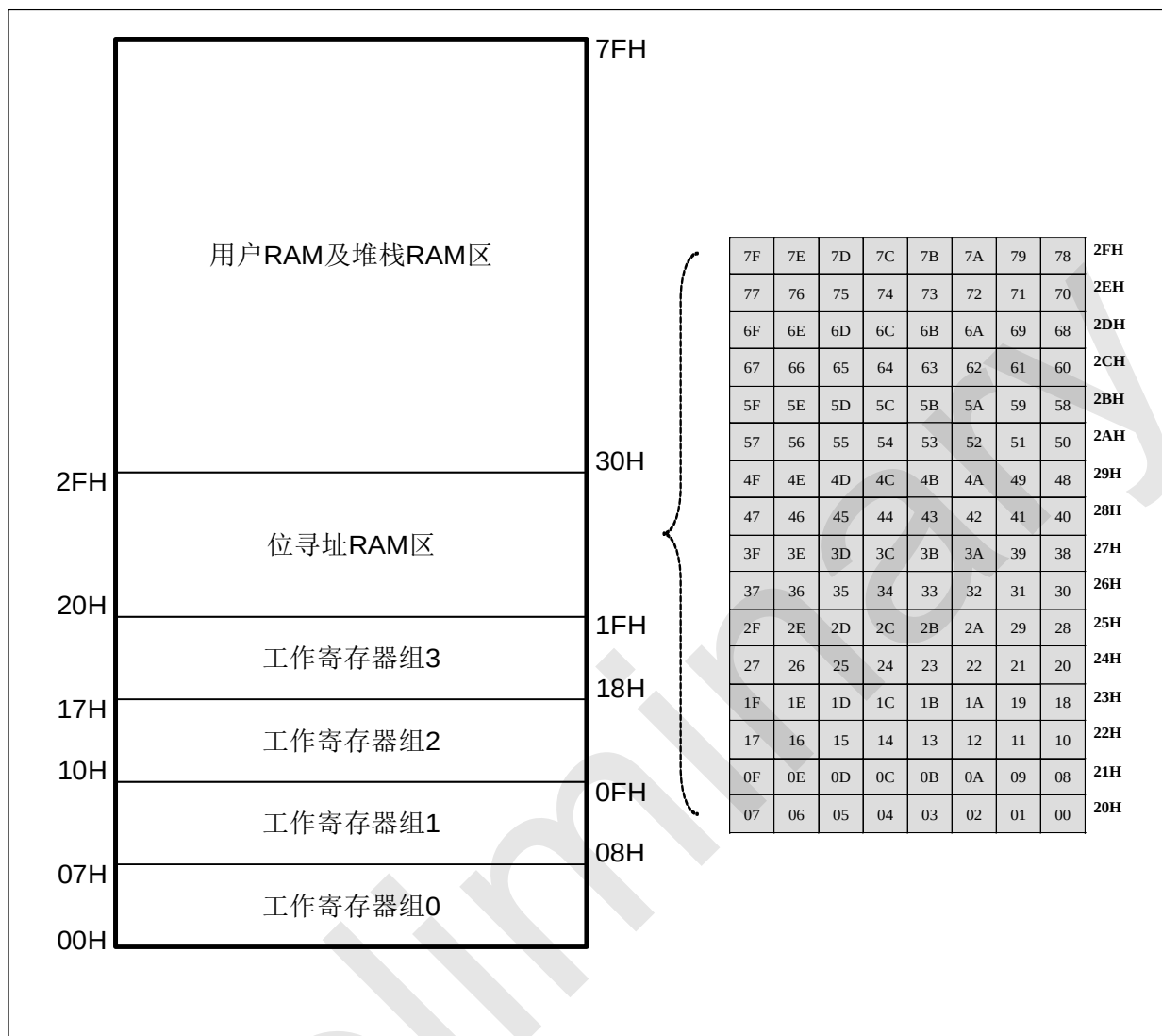
SRAM 结构图
