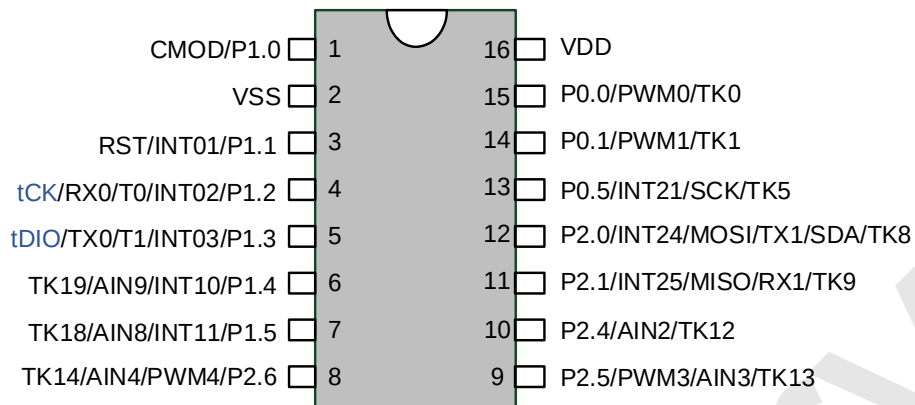
SOP16 管脚配置图
