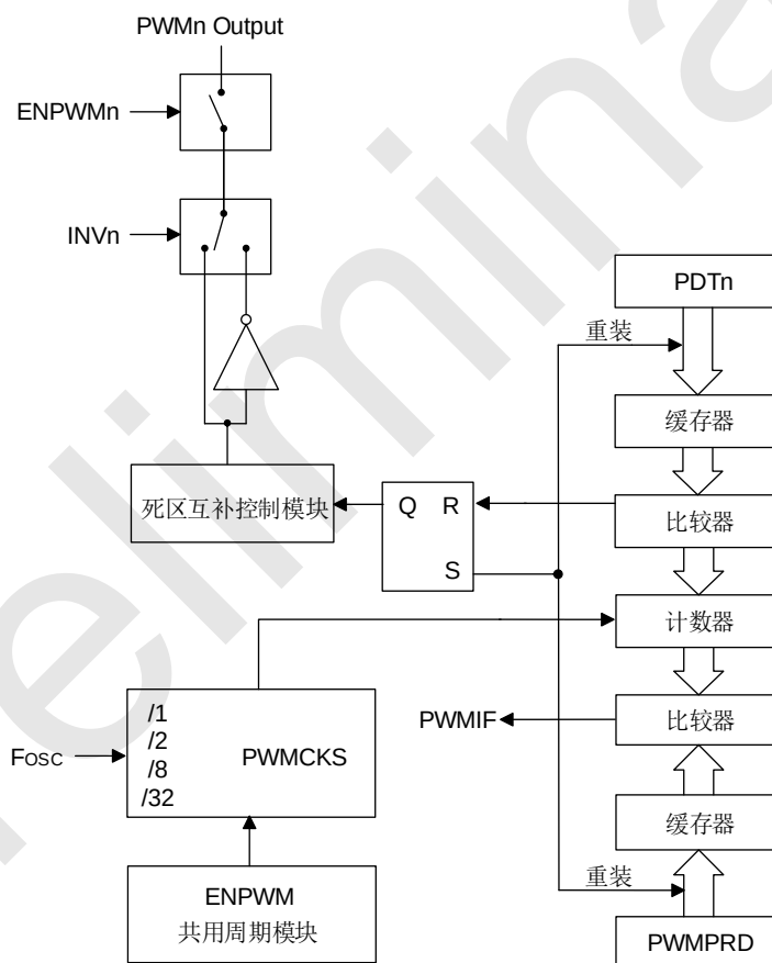
SC92R348 PWM 结构框图
